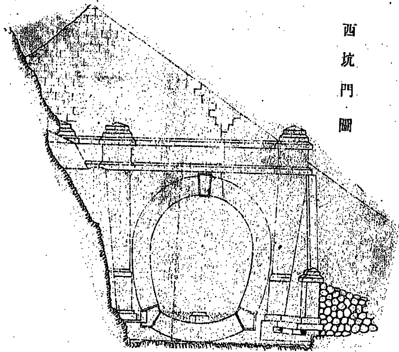
改築設計圖
